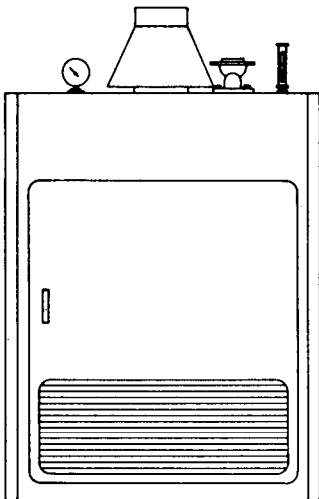
Alzado frontal
