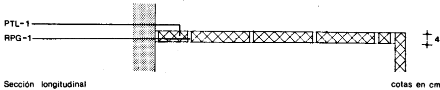
Sección longitudinal
