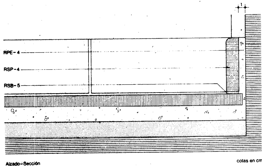
Sección B-B
