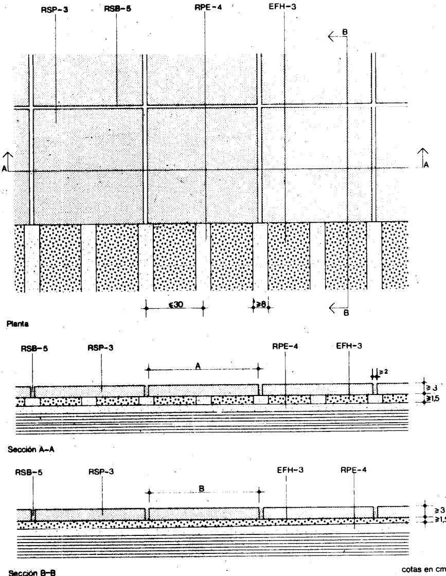
Sección B-B
