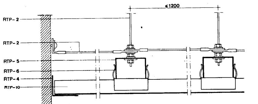
Sección longitudinal
