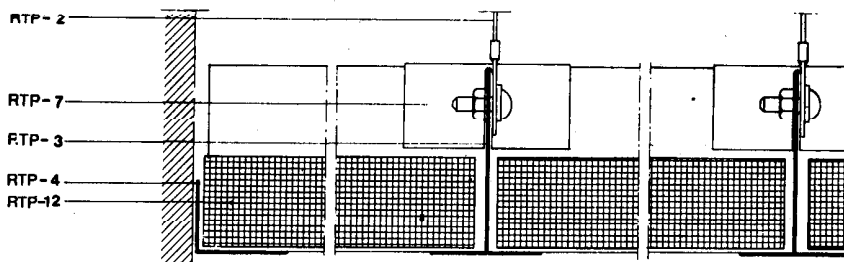
Sección transversal
