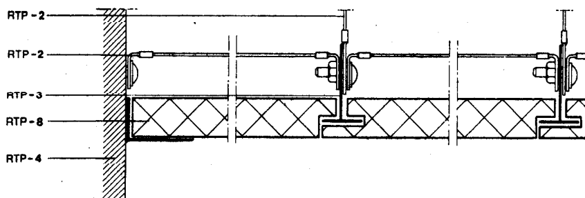
Sección transversal
