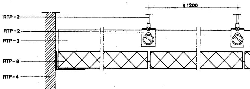
Sección longitudinal
